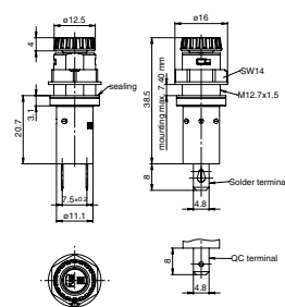
IP67 / Varianten Fingergrip 3101.0125 und 3101.0325
