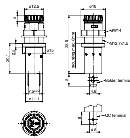
IP40 / Varianten Fingergrip 3101.0025 und 3101.0225
