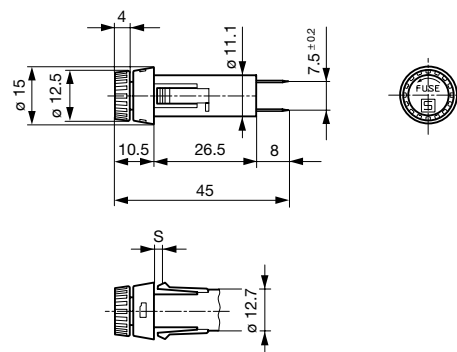
Varianten Fingergrip 3101.0035, 3101.0235, 3101.0036 und 3101.0336 s = Plattendicke (siehe Variantentabelle)
