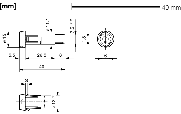
Varianten 3101.0030, 3101.0230, 3101.0031 und 3101.0331 s = Plattendicke (siehe Variantentabelle)
