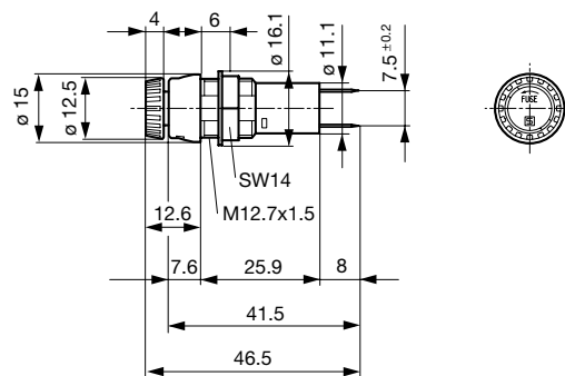
IP67 / Varianten Fingergrip 3101.0115 und 3101.0315
